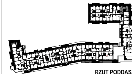
RZUT PODDASZA KONDYGNACJA 2
